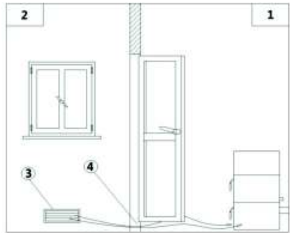
Fig. 7 - Afluencia del aire indirecta
