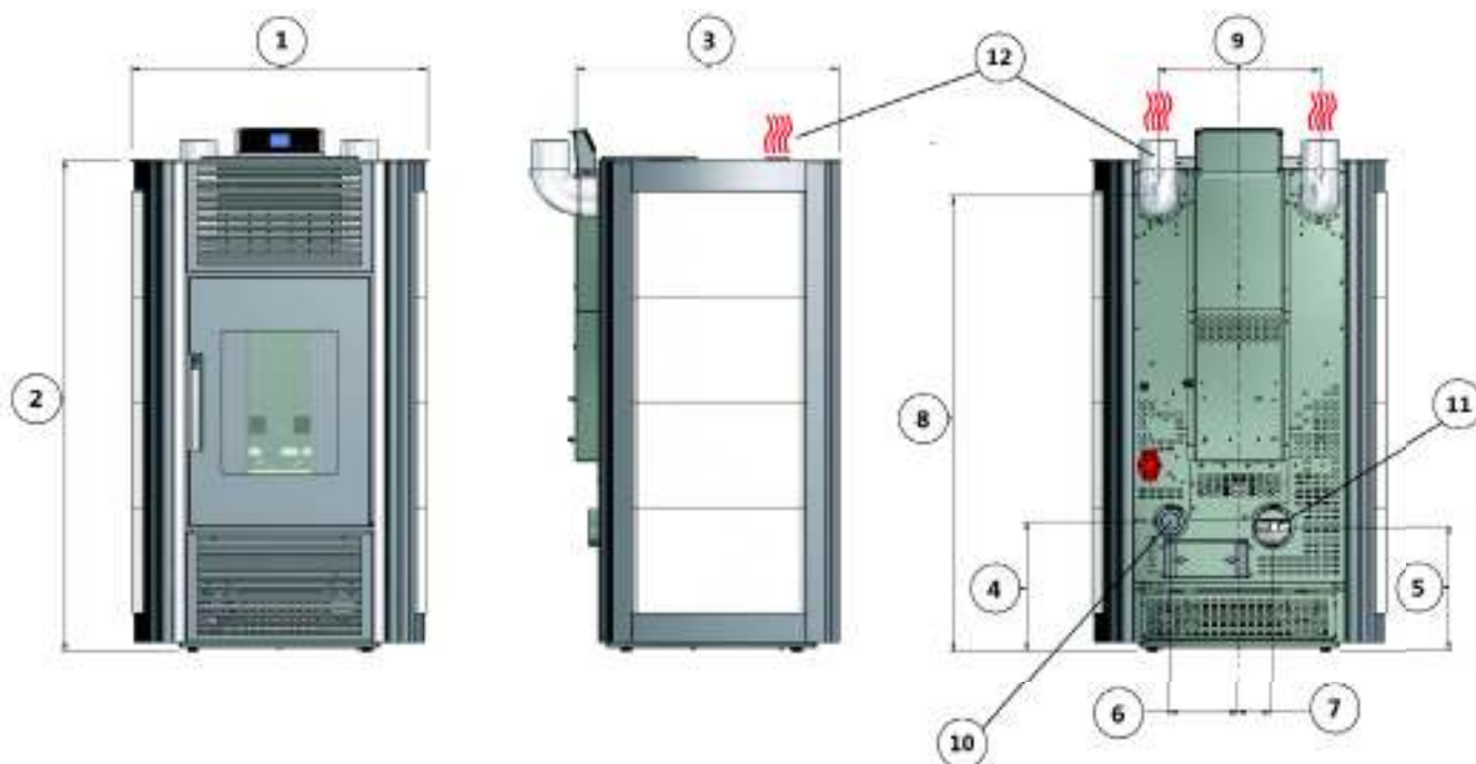
Fig. 11 - Dimensiones generales
